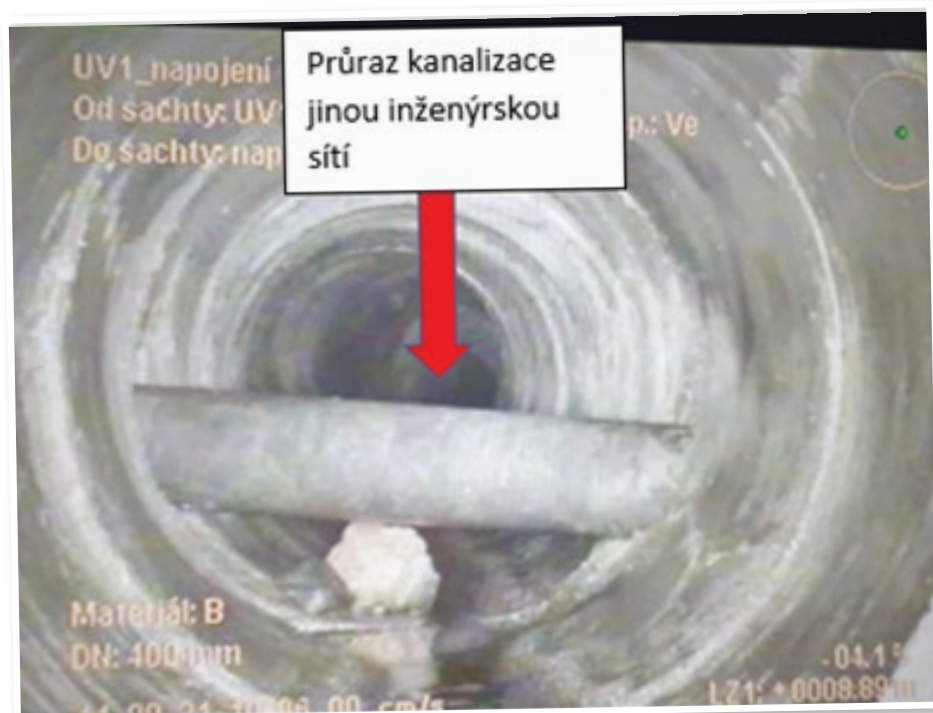
Průraz stávající betonové kanalizace jinou sítí (po provedení sondy zjištěno, že se jedná o kabely telefonu v ocelové chráničce)
