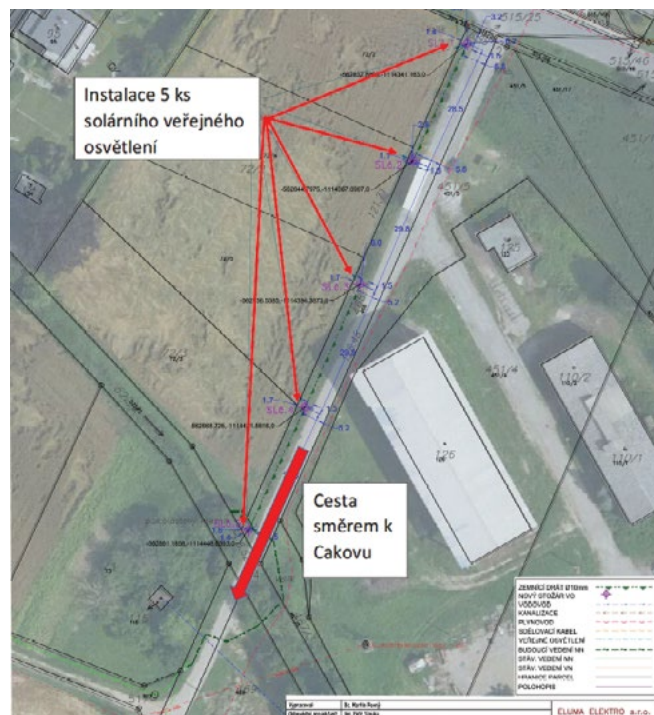
Schéma umístění 5 ks solárního veřejného osvětlení směrem k Cakovu.
